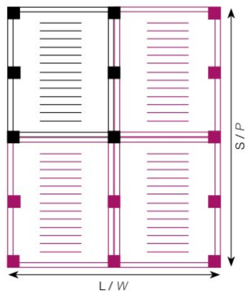
MODULO QUADRUPLO ACCOPIATO IN PROFONDITÀ Dimensioni massime: L 1000 x S 2020
