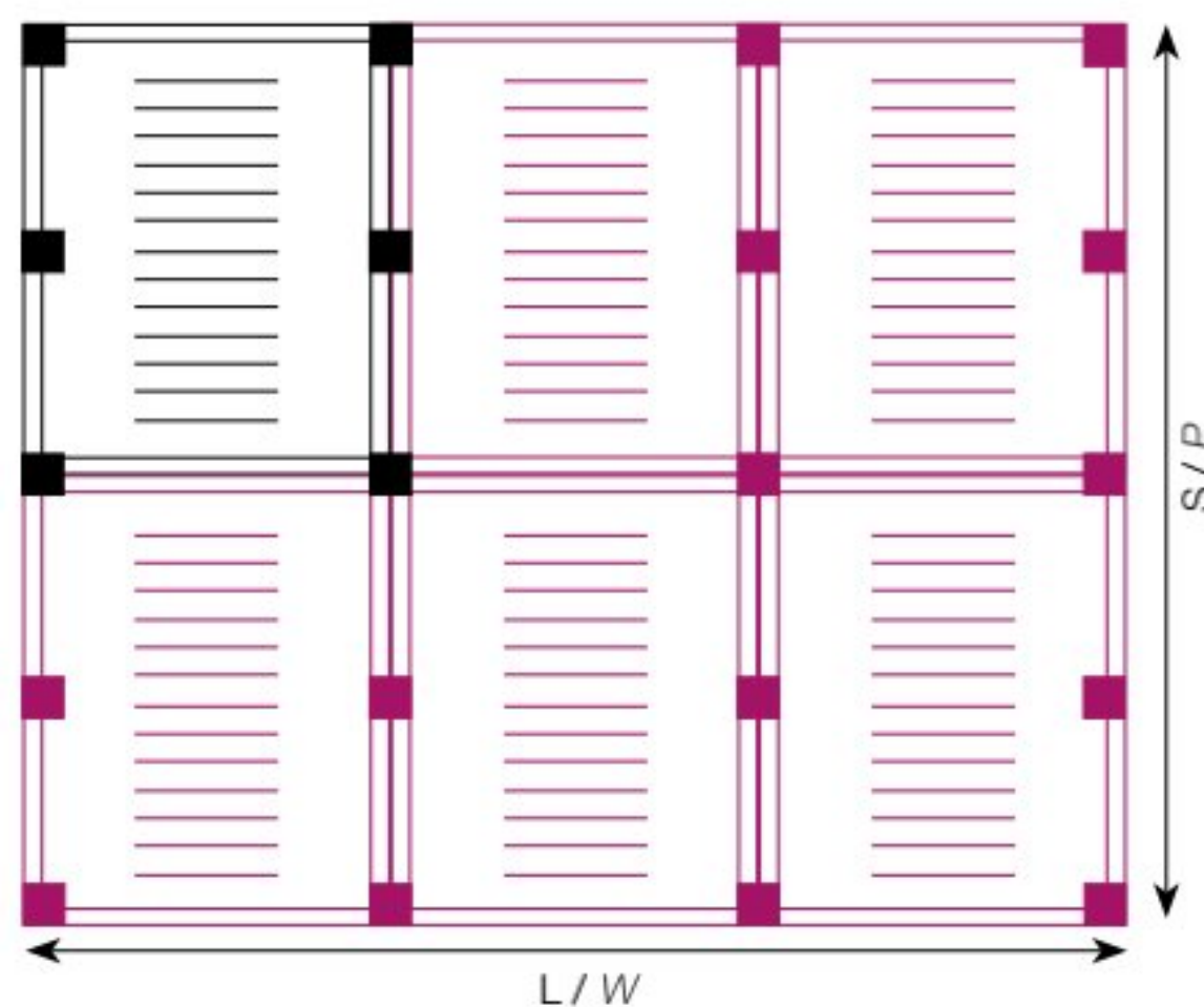
MODULO SESTUPLO ACCOPIATO IN PROFONDITÀ Dimensioni massime: L 1500 x S 2020
