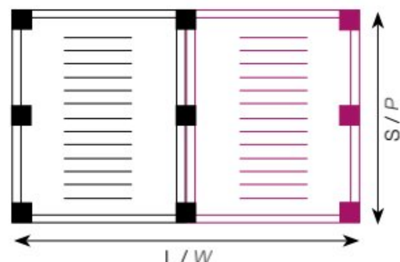
MODULO DOPPIO ACCOPIATO IN LARGHEZZA Dimensioni massime: L 1000 x S 1010
