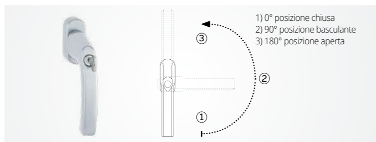
FERRAMENTA TBT (TILT BEFORE TURN) inclinare prima dell'apertura - protezione con chiave contro l'apertura totale della finestra
