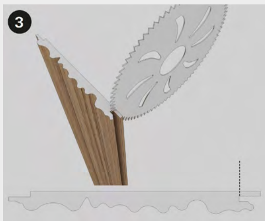
Tagliare il nuovo pannello come mostrato in figura, eliminando il labbro dell'incastro "femmina".
